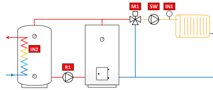
7. Circuit 1 et eau chaude sanitaire vanne ouverte
