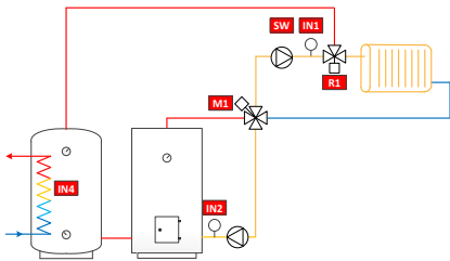
12. Circuit 1, priorisation de l'eau de retour et eau chaude sanitaire vanne ouverte
