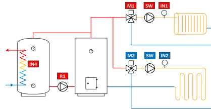
8. Circuit 2 et eau chaude sanitaire vanne fermée
