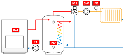
5. Circuit 1 et cheminée/poêle
