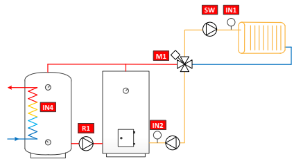
11. Circuit 1, priorisation de l'eau de retour et eau chaude sanitaire vanne fermée
