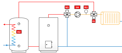
7. Circuit 1 et eau chaude sanitaire vanne ouverte
