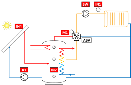
14. Vanne bivalente et capteur solaire
