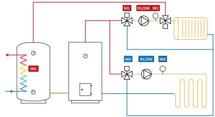
9. Circuit 2 et eau chaude sanitaire vanne ouverte
