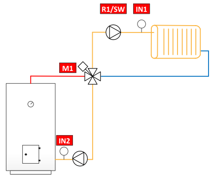
11. Circuit 1, priorisation de l'eau de retour et eau chaude sanitaire vanne fermée
