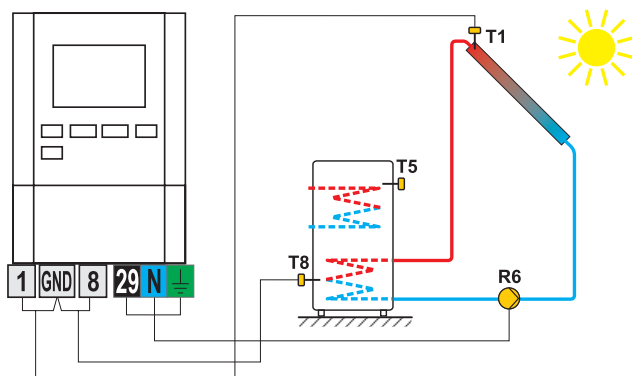
Schéma 1- Chauffe-eau sanitaire
