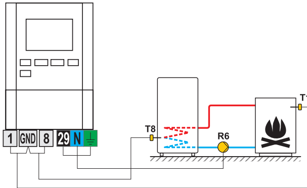
Schéma 1- Chauffe-eau sanitaire
