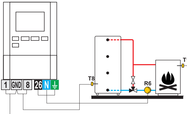
Schéma 2 - Ballon
